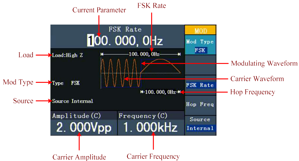
Abb. 0-19: Die Benutzeroberfläche der FSK
